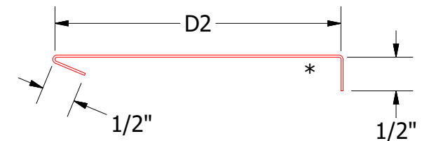
Head Angle Trim DWA690: D2= 4 1/4" DSA690: D2= 5"
