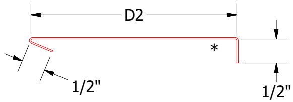
Head Angle Trim DWA690: D2= 4 1/4" DSA690: D2= 5"
