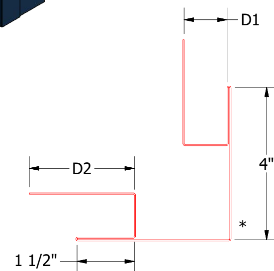
Outside Corner Post DWA602: D1 = 1 1/8", D2 = 2 3/4" DSA602: D1 = 1 7/8", D2 = 3"
