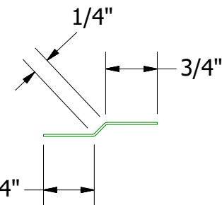
VLA975 - Joggle Cleat
