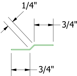
VLA975 - Joggle Cleat
