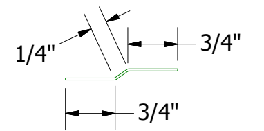
VLA975 - Joggle Cleat
