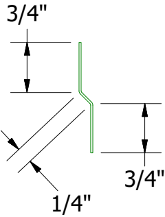
VLA975 - Joggle Cleat
