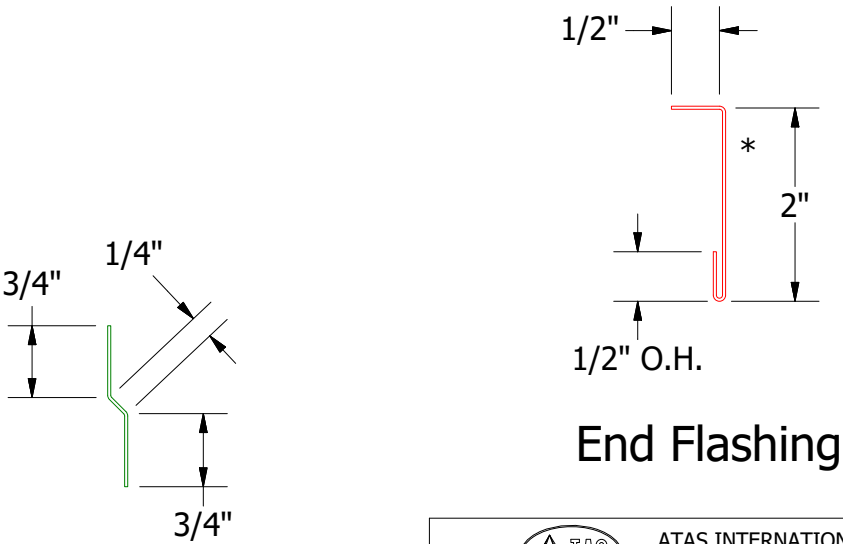
VLA975 - Joggle Cleat
