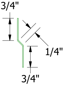
VLA975 - Joggle Cleat
