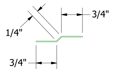
VLA975 - Joggle Cleat
