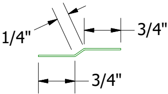
VLA975 - Joggle Cleat
