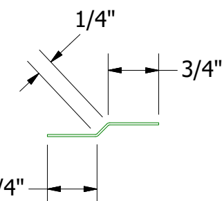
VLA975 - Joggle Cleat
