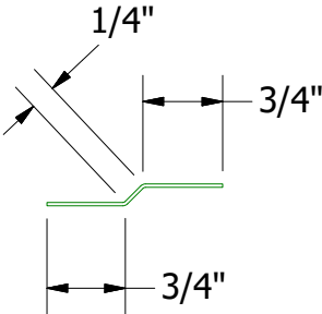
VLA975 - Joggle Cleat
