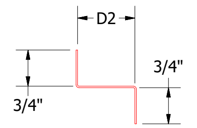
Z Closure D2=1 3/16" D2=1 15/16"
