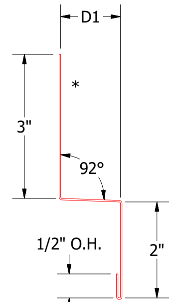
Head Trim DWA550: D1=1 1/4" DSA550: D1=2"
