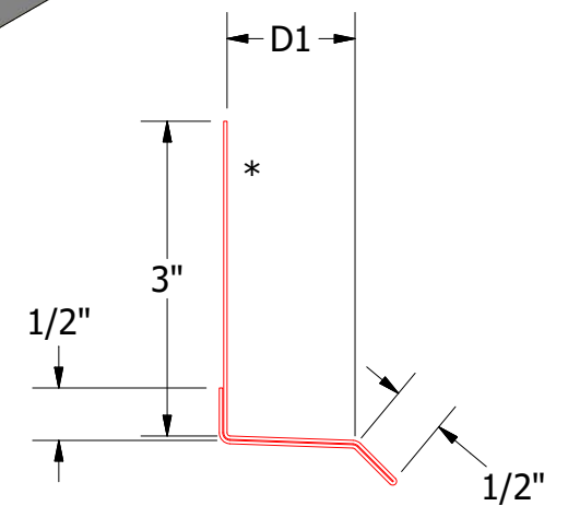
Base Trim - Standard DWA661: D1 = 1 1/4" DSA661: D1 = 2"
