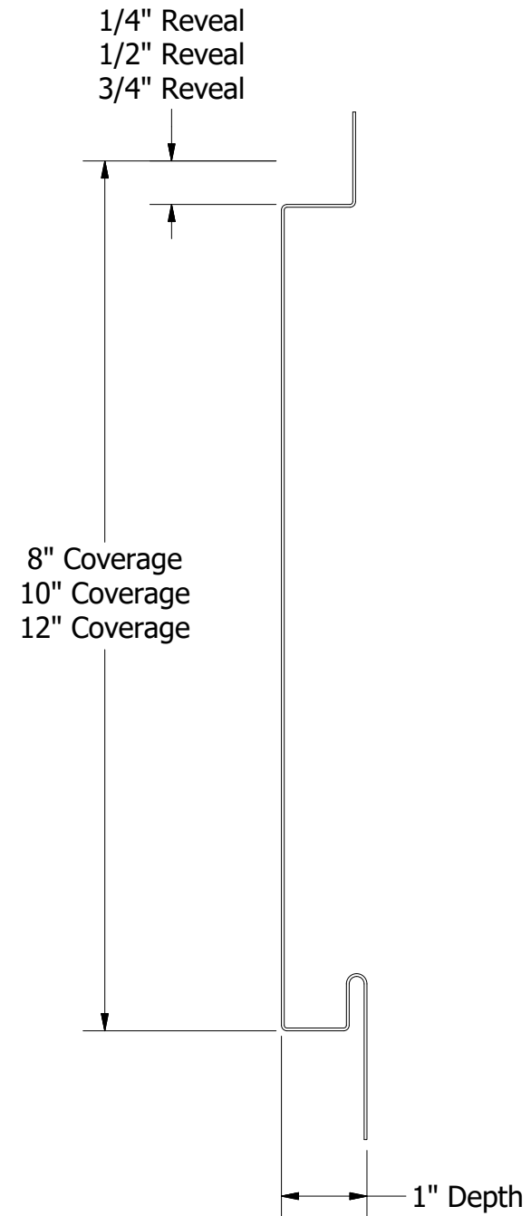
Section A-A
