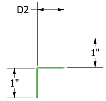
Support Z DWA681: D2 = 1" DSA681: D2 = 1 5/8"
