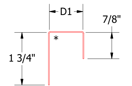
J Closure DWA270: D1 = 1 1/8" DSA270: D1 = 1 7/8"
