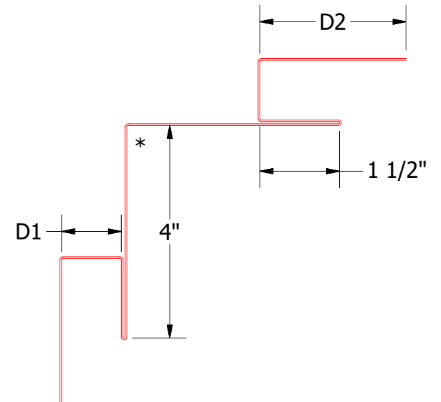
Inside Corner Post DWA601: D1 = 1 1/8", D2 = 2 3/4" DSA601: D1 = 1 7/8", D2 = 3"
