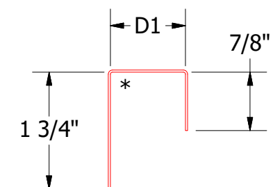
J Closure DWA270: D1 = 1 1/8" DSA270: D1 = 1 7/8"
