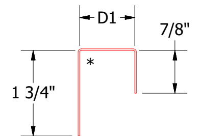
J Closure DWA270: D1 = 1 1/8" DSA270: D1 = 1 7/8"
