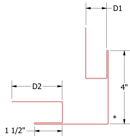
Outside Corner Post DWA602: D1 = 1 1/8", D2 = 2 3/4" DSA602: D1 = 1 7/8", D2 = 3"
