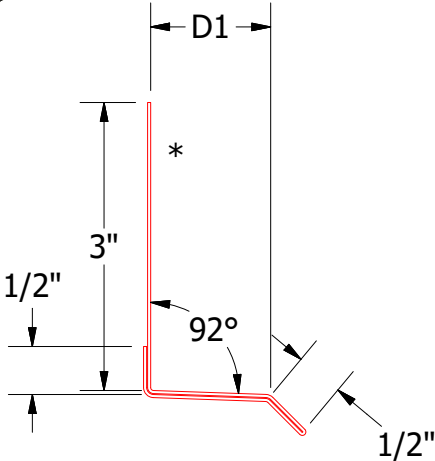
Base Trim - Standard DWA661: D1 = 1 1/4" DSA661: D1 = 2"
