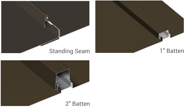
2" Batten
