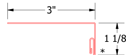
VSA119 - Snap J Base
