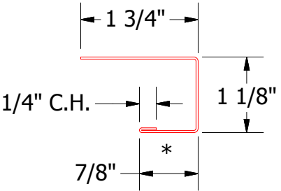
VSA118-J Channel
