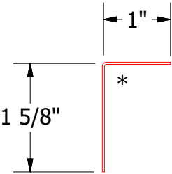
VSA680 - Angle Trim
