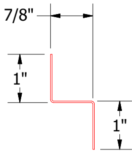
VSA681-Support Z
