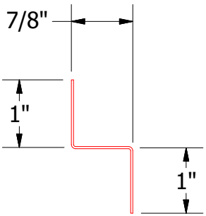
VSA681-Support Z
