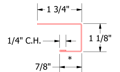
VSA118-J Channel
