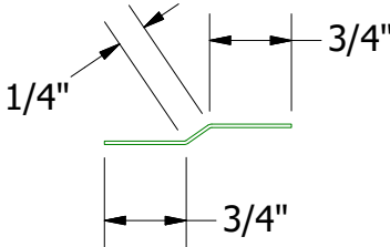
Joggle Cleat
