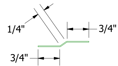
Joggle Cleat
