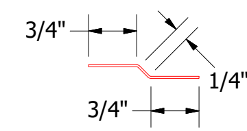
Joggle Cleat
