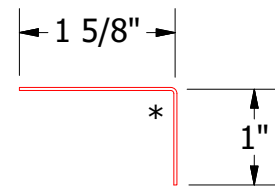
VSA680 - Angle Trim
