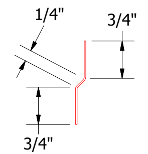
PCA975-Joggle Cleat
