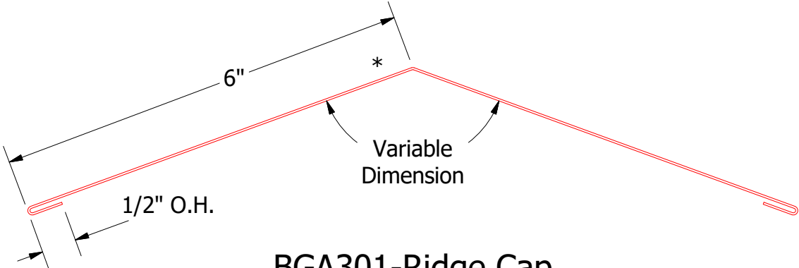
BGA301-Ridge Cap
