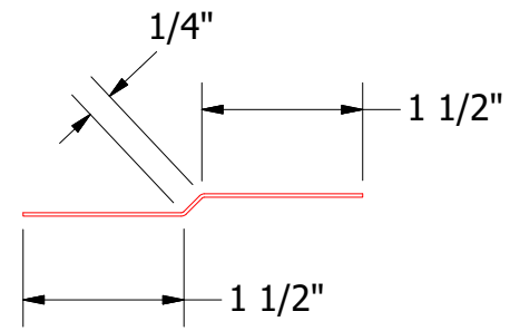
FLA975-Joggle Cleat (NTS)
