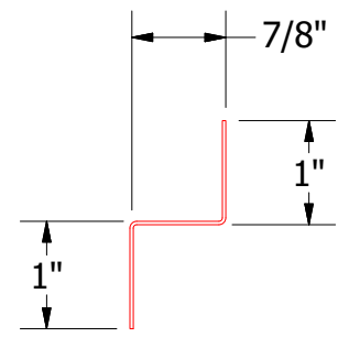
VSA681-Support Z
