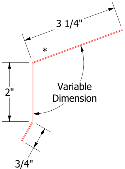
SCA175-Drip Edge
