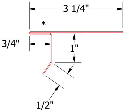
HSA112-Drip Edge
