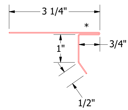
HSA112-Drip Edge
