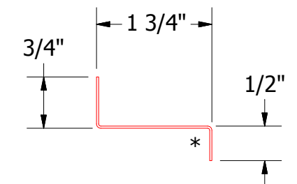
Jamb Angle
