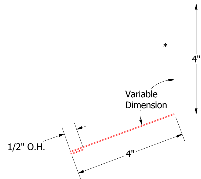
HBA502-Headwall Trim
