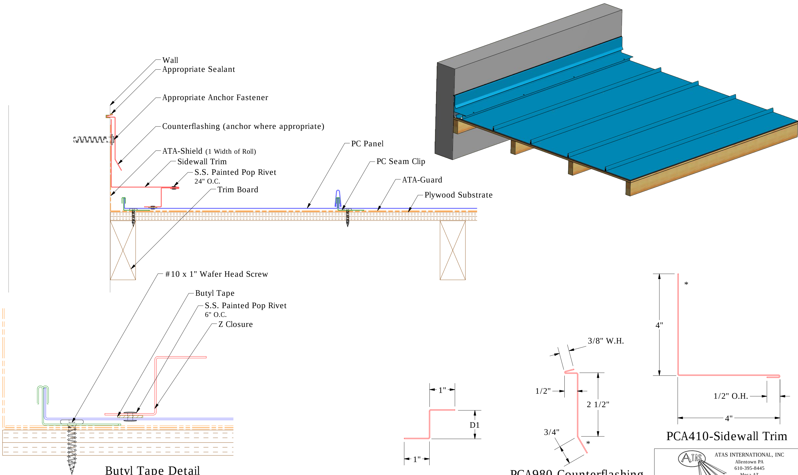
Z Closure PCA910 - 1" Seam and 1" Batten D1=1 1/8" PCA912 - 2" Batten D1=2 1/8"
