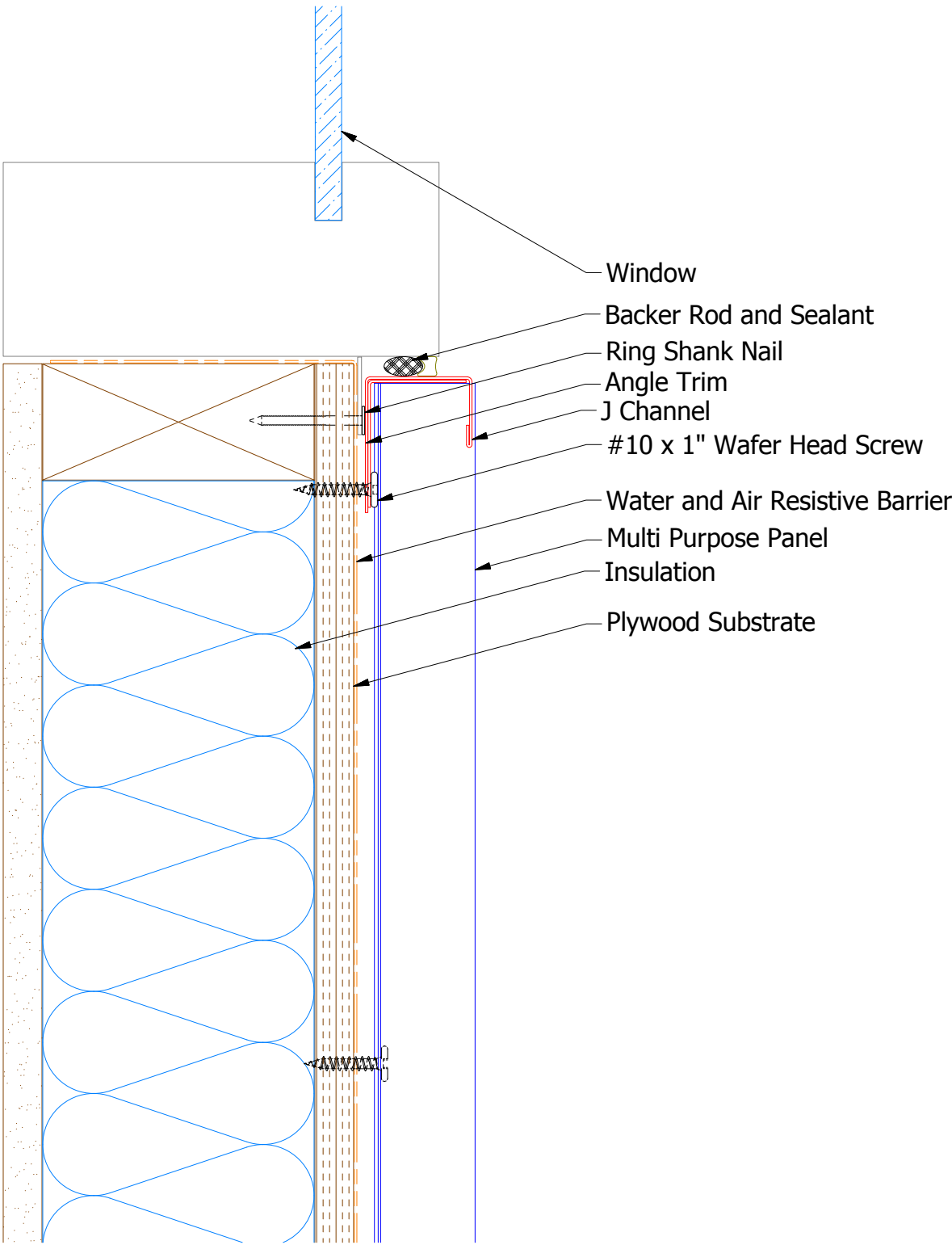
MPA680 - Angle Trim
