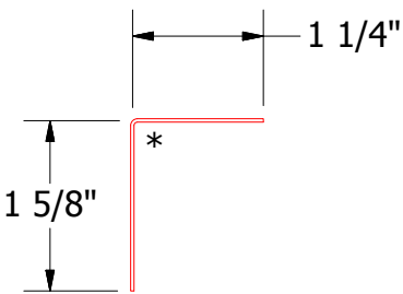
MPA680 - Angle Trim
