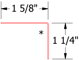
MPA680 - Angle Trim
