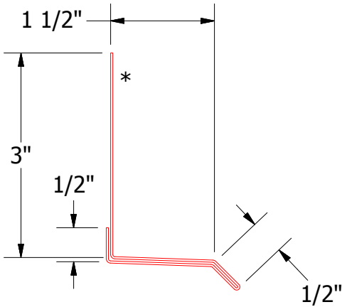
MPA661 - Base Trim
