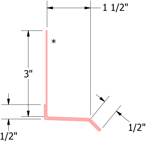
MPA661 - Base Trim
