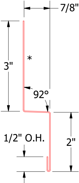
MFA550 - Head Trim
