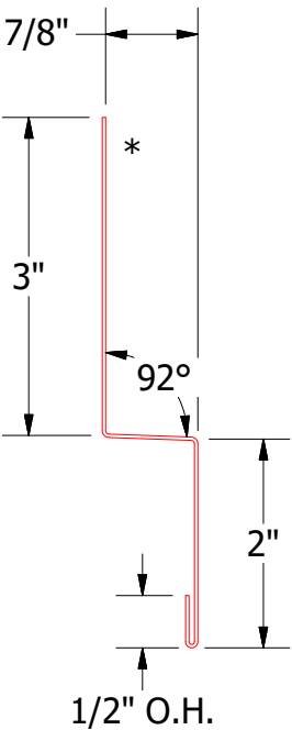
MFA550 - Head Trim
