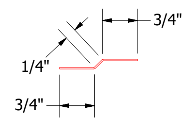
MDA975-Joggle Cleat (N.T.S.)
