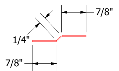
MDA975-Joggle Cleat (N.T.S.)
