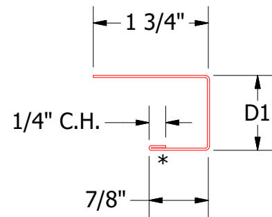
J Channel DWA118: D1=1 1/8" DSA178: D1=1 7/8"
