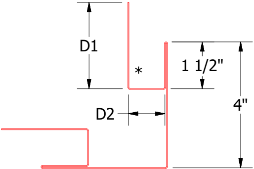
Outside Corner Post DWA602: D1= 2 3/4"; D2= 1 1/8" DSA602: D1= 3"; D2= 1 7/8"
