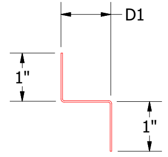
Support Z DWA681: D1= 1" DSA681: D1= 1 5/8"
