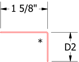
Angle Trim DWA680: D2= 1 1/8" DSA680: D2= 1 3/4"
