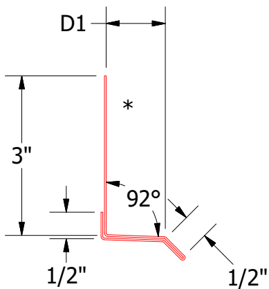
Base Trim DWA661: D1= 1 1/4" DSA661: D1= 2"
