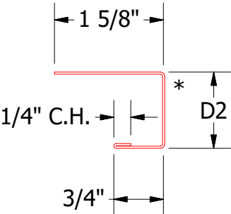
J Channel DWA118: D2= 1 1/8" DSA178: D2= 1 7/8"
