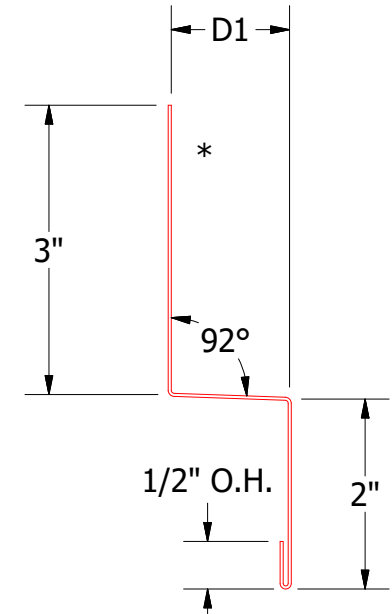
Head Trim DWA550: D1= 1 1/4" DSA550: D1= 2"
