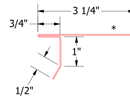
HLA112-Drip Edge
