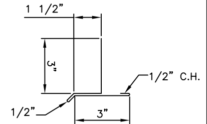
MPA662 'T' SILL TRIM
