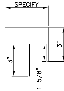
JAMB TRIM
