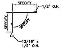
SILL TRIM - MPA673
